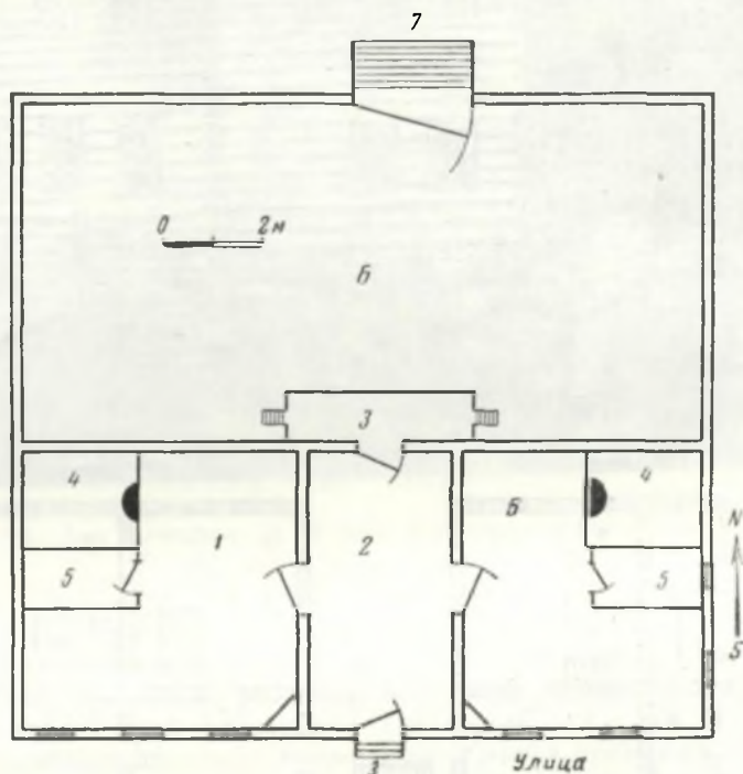
Рис. 65. Старинная планировка в трехраздельном доме с маленьким окном в боковой стене (с. Усть-Кулом Усть-Куломского района Коми АССР).
