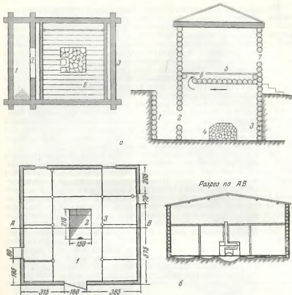
Рис. 76. Планы и разрезы овина и риги:
