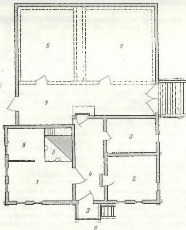
Рис. 61. Трехраздельный дом старого типа (д. Усть-Кожва Кожвинского района Коми АССР).
