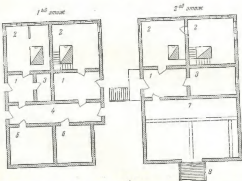
Рис. 64. Двухэтажный дом (с. Усть-Уса Коми АССР).
