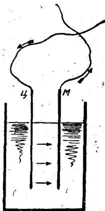
14 rıis. Galvaničeskəj element. Tatən ximičeskəj eņergija pə-rə električeskəj eņergijaə.
