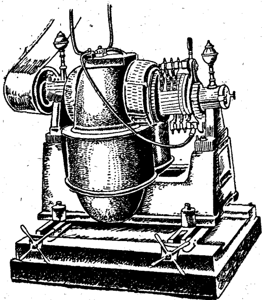
15 ris. Dinamomasina. Sььn seditšə električestvo tok.
