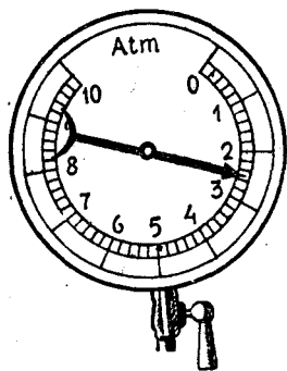
4 ris. Metaliѣ керѣм manometra, kѣdaѣn para koѣollezнѣн merajtnѣнѣ нѣрѣstѣmsѣ.
