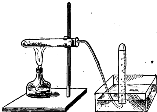
10 ris. To kəz kolə sedtəny kislərod.
