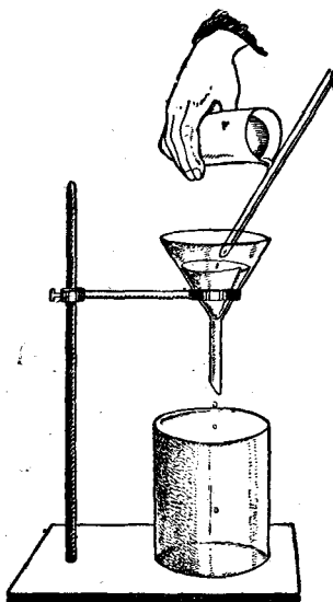
7 ris. To kьz vəđokət kolə kiřьňь filtraə va.
