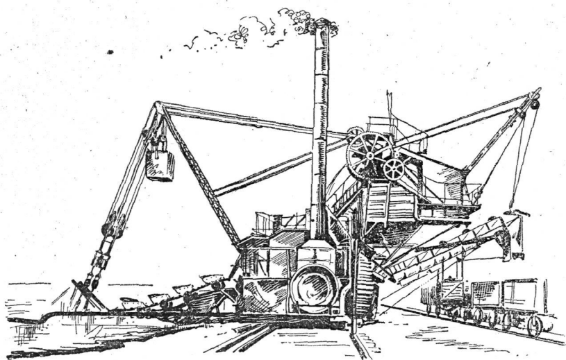
23. Əkskavatorrezən sov sedtəny.
