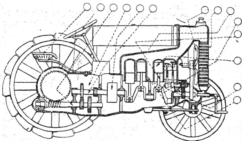
92. Kъz kerъm traktor.
