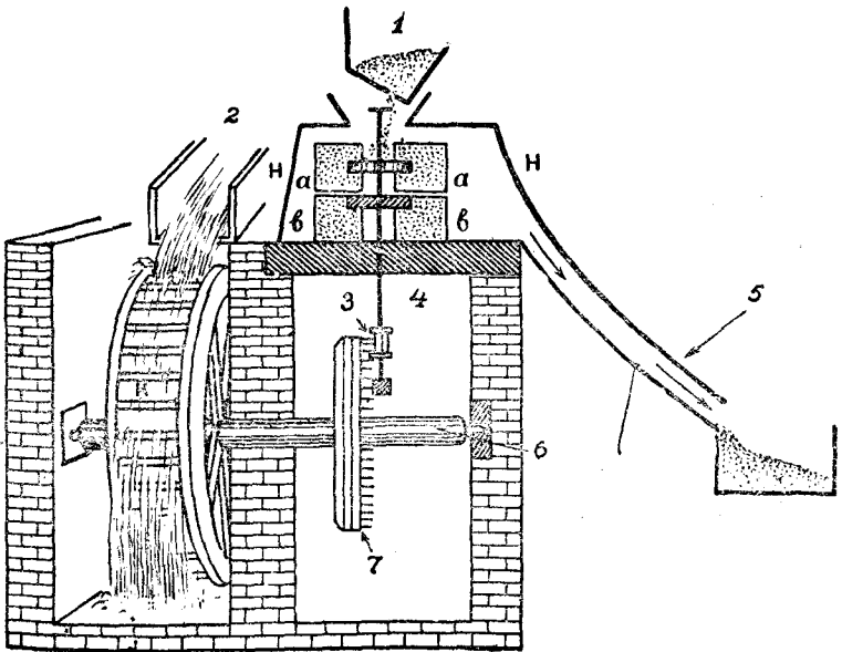
Kыз kerēma va vylēn uzalan meļņica (sxema).
