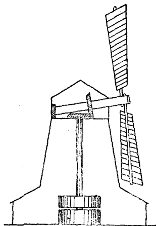
Vətrjak sxema.
