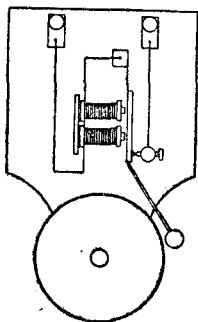
Електрическәй звонок.
