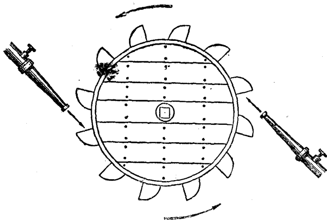
Kəz uzalə para tutsinalən koļoso (схема).
