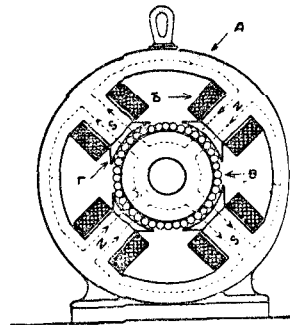
Динамомасина vundьstəma. A— stanina. S — elektromagnittez I — šərkərt elektromagnitlən mьtčişəma B. — šərkərt vьləə kač-təma mednəj provka
