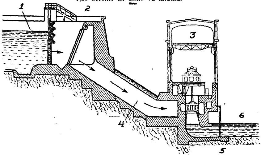
Cidrostancija dol vundüstäma. 1. Kanal'n sulalõ va 2. Plotina. 3. Stancija kerku. 4. Va lezan truva. 5. Va kõskan truva. 6. Juõn sulalõ va.
