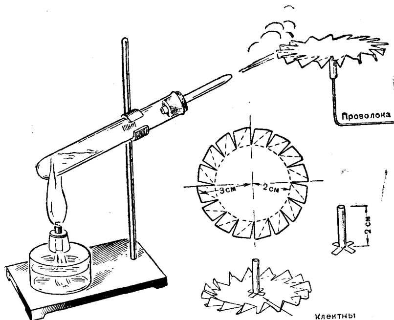
Рис. 25. Паровой турбиной бумажной модель.
