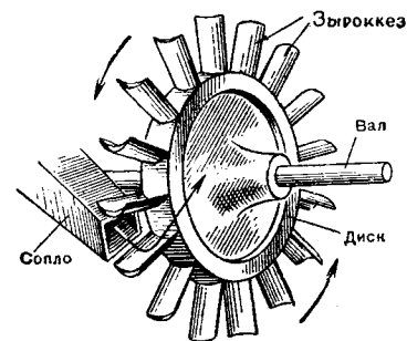
Рис. 24. Паровой турбина.
