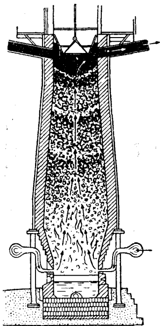
Рис. 74. Доменнöй гор (вундыштöмөн).
