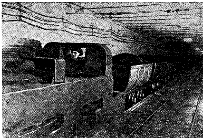
Рис. 67. Электровоз.
