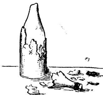
Рис. 13. Йы жугдис бутылка.
