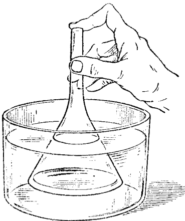
Рис. 30. Воздух занимайтö места: ва оз пыр воронкаас.
