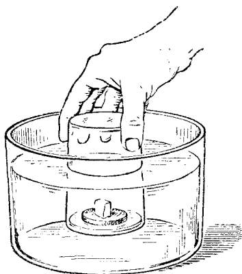
Рис. 31. Воздух занимайтӧ места: ва оз пыр стаканас.
