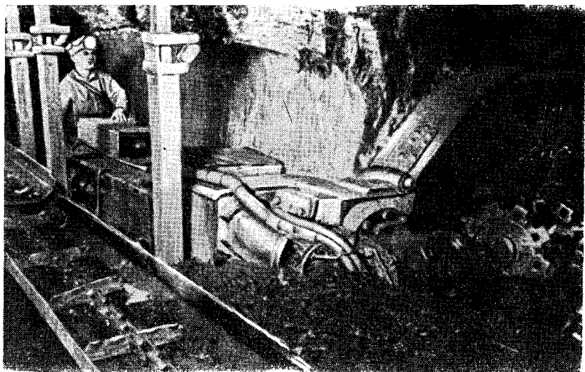
Рис. 66. Угольной комбайн.
