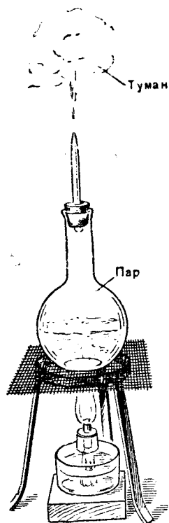
Рис. 8. Валöн пизьöм. Пар нетыдалан.
