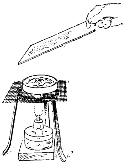
Рис. 80. Почваын эм ва.
