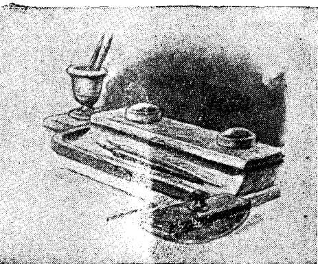
Рис. 55. Мый керөны мраморись.
