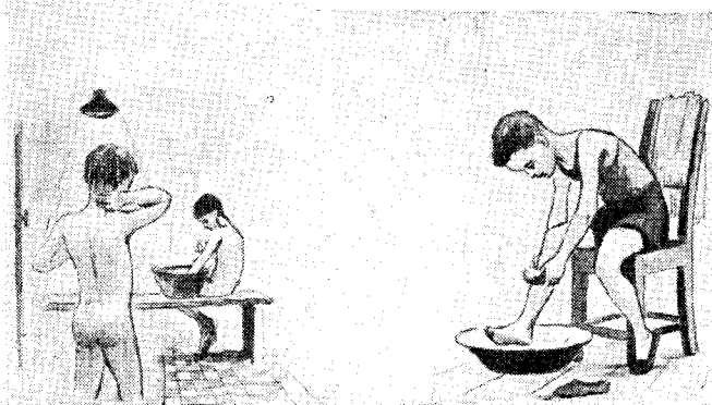
Рис. 95. Мый колө керны, медбы тело вөлі сөстөм.
