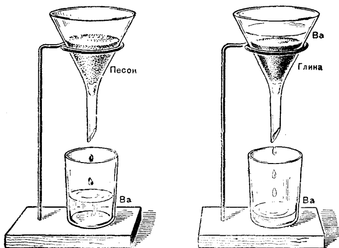
Рис. 52. Песок пыр ва йиджө бура, а глина пыр ва йиджө умөля.
