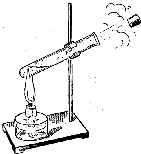
Рис. 19. Пар тойыштіс пробиркаыс пробкасö.
