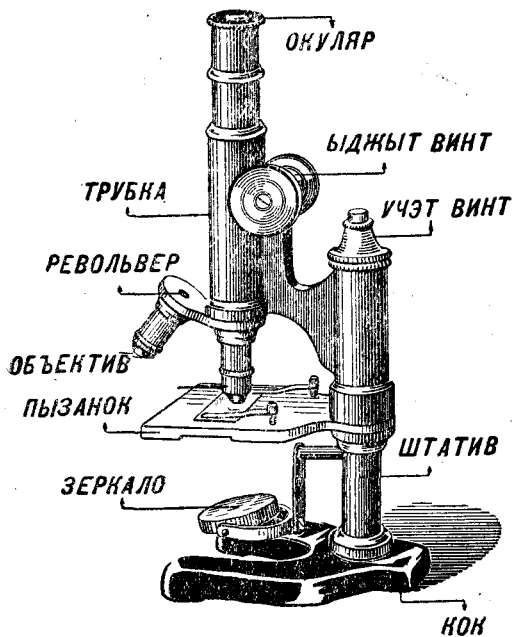
Рис. 68. Микроскоп.
