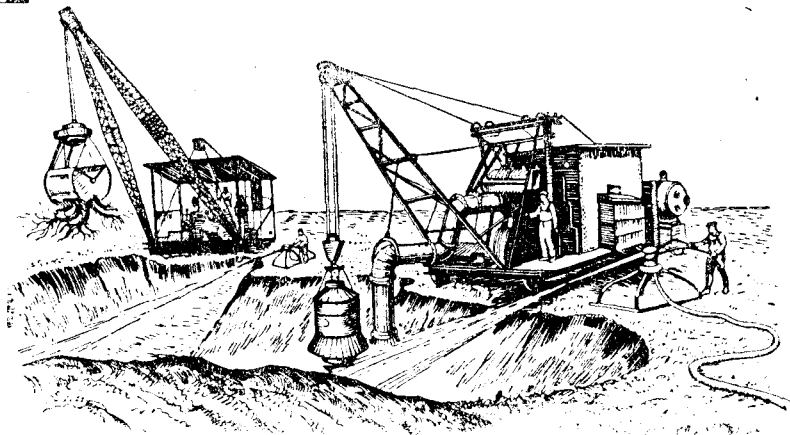
Рис. 13. Машинаэзён торф шедтём.
