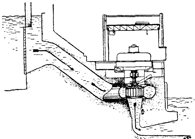
Рис. 33. Кыдз сувтӧтӧм ваа турбина Днепрогӛсын.
