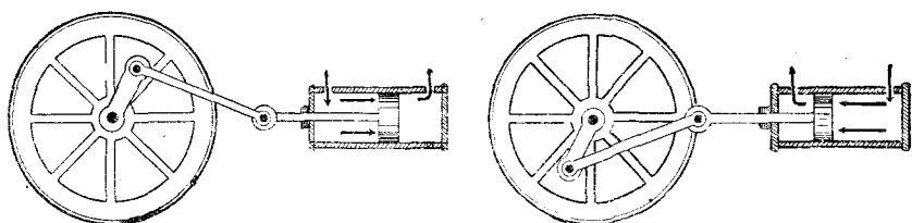
Рис. 34. Кызды пар нырыштё поршень вылё да бергётё колесо.
