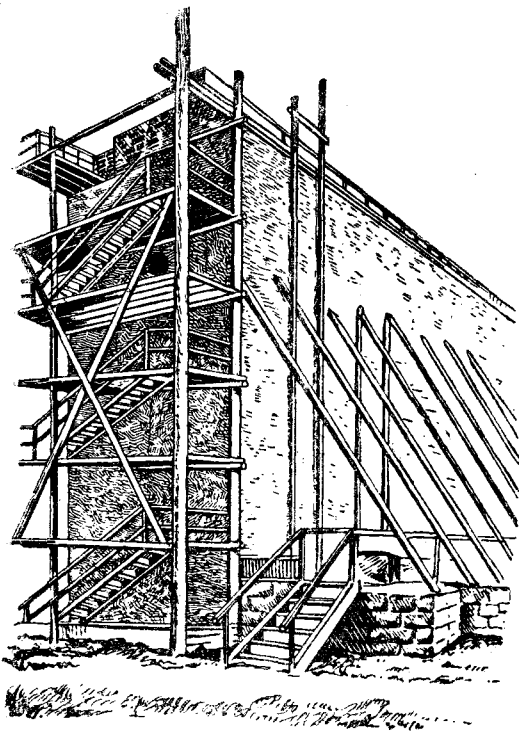
Рис. 10. Градирня.
