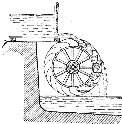
Рис. 32. Ваа колесо (наливнöй).
