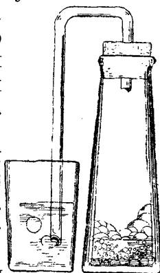
Рис. 49. Углекислöй газ шедтöм.
