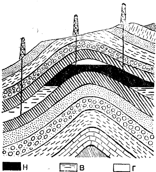
Рис. 20. Муын нефтьлөн куйлём; Н—нефть, В—ва, Г—газ.
