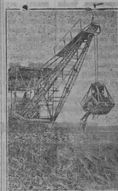
В Балахне (Нижегородск. губ.) стро- ится новая электростанция, которая будет работать на торфе. На снимке: механическая кормовка пней на торфоразработках электро- станций.
