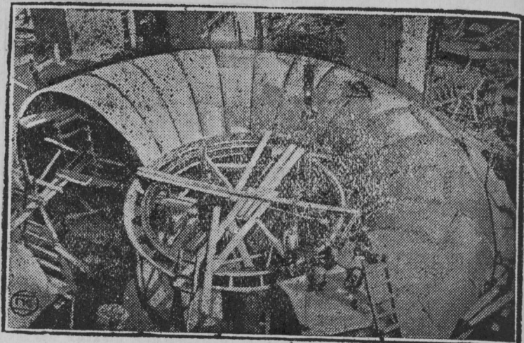
На снимке: Монтаж турбины.
