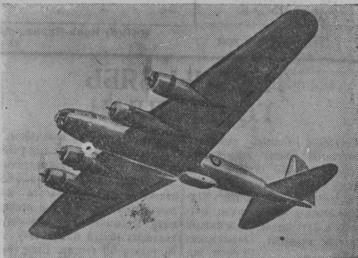
Американский бомбардировщик «Летающая крепость» на службе в английских воздушных силах. Скорость бомбардировщика превышает 300 миль в час, дальность полета 3500 миль, потолок 36000 футов, размах крыльев 105 футов, длина 70 футов, высота 15 футов. Бомбовый груз составляет несколько тонн.
