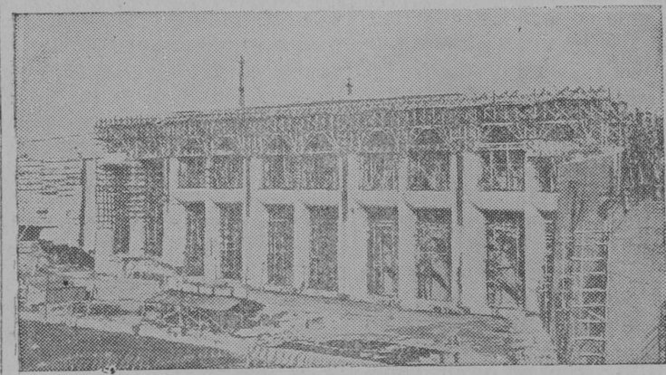
На строительстве Рыбинского гидроузла. На снимке: Общий вид железобетонной плотины через реку Волгу с верхнего бьефа. Фото М. Королева. Бюро-клише ТАСС.
