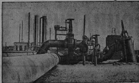
На снимке: Первая станция подземной газификации угля в Донбассе. Фото В. Небылицкого. Бюро-клише ТАСС.
