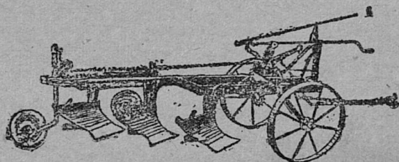
16 серп. Пинчер маркаа куім корпуса тракторнөј Сакка плуг. Лыпасјасыс петкөдлөвы: 1 — автоматыскөд јитчан сает, 2—көлөсајасө ладмөдан рычаг.
