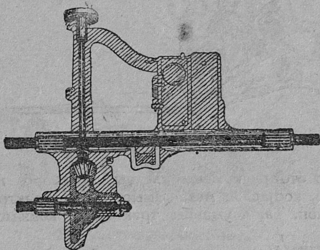
42-а серп. Ыцкан машиналөн рамаыс. Шугалаас пунктөма вал, вал өтар помас коническөј зубчатка, мөдар помас кривошип.
