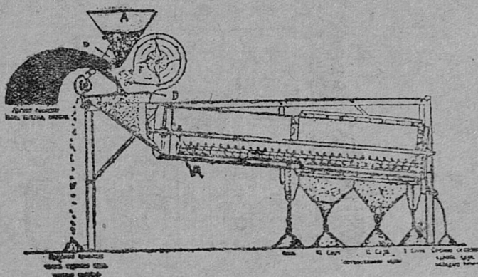
72 серп. Кыквеса тріер шөрөдыс вундөмөн. А—көш, Б—туе вешталаи валік, В—пөж, Г—вентилатор. d—тріера циліндр.
