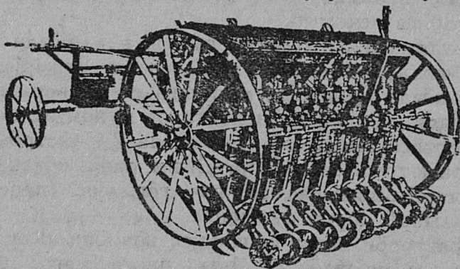
35 серп. Öглаалöм (комбинирүлтöм) көзән Сопникјас бөрсөыс вöтчöны гөгыл-јас, көдјас мусö топöдöмы.
