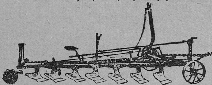
17 серп. Тракторнөј лушцілнык
