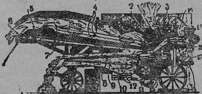
60 серп. Сложнөй молотылака шөрвундасөдыс виқөдөмөн. Лыднјасыс ге көдлөны: 1—көлта пукталан воронка, 2—вартан барабан, 3—барабан увт, 4—іңаспыркөдан, 5—седтөда іңаспыркөдан, 6 веекөдлаан решета, 7—горувса пөв, 8—грехот, 9 ісковтан доска, 10—јікі грехот, 11—вентилатор, 12—пож, (возсө виқөд 61 серпасыс)
