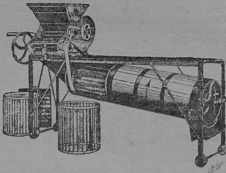
71 серп. Триер-куколеотборник.
