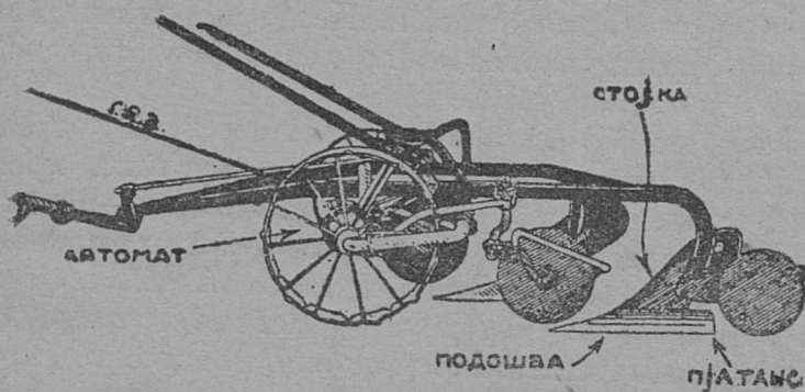
14 сери. Америкаса тракторноҗ плуг. Бевдорас—веекыд- ладорсааныс—гөрөмлааҥсааныс — виҗөдөмөн; увдорас—гө- рөмлааҥсааныс виҗөдөмөн.
