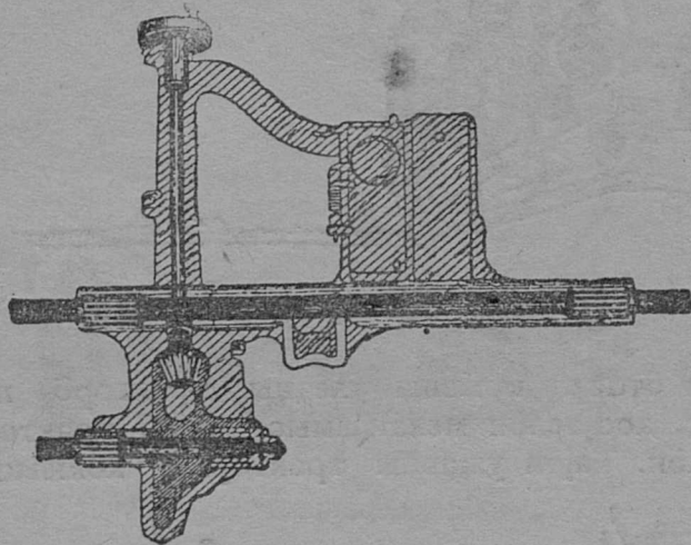
42-а серп. Ышқан машиналөң рамаыс. Шугалаас пунктөма вал, вал өтар помас коническөј зубчатка, мөдар помас кривошіп.
