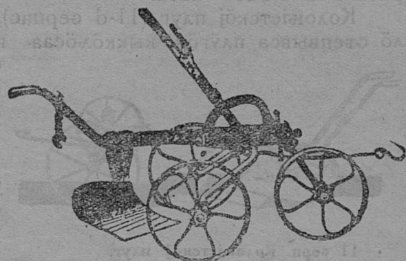
9 серп. Өтө вөлөн кыскалана рамаа плуг
