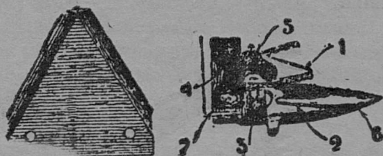
39 серп. Пурта пластинка (шужалаас) да вундан аппарат (веекылаас). Лыдпасжасыс петкөдлөны: 1—пурта пластинка, 2—пластинкаыс чукас 3—пурта полосаыслөн удор горбыс, 4—мыжсан пластинка, 5—зелөдөм лапөд, 6—чун, 7—чун- кутөд брус.
