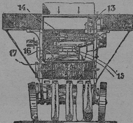
61 серп. Сложнөј молотїаквалөн шөрвундас. Лыдпасјасыс петкөдлөны: 13—елеватор, 14—шас-талка, 15—грохот, 16—пөж, 17—сортірујтан.
