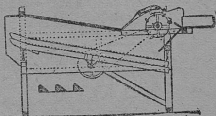
53 серп. Гысегь сеталан да ізас-пыркөдана вартан машиналөн шөр-вундасыс. Пыщкас петкөдлөма пу брусјасыс модасө.
