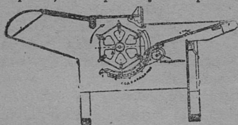
54 серп. Улысан сеталан моло-тилкалөн шөрвундасыс. (пөчөма „Краснаја Ывезда“ заводуын,
