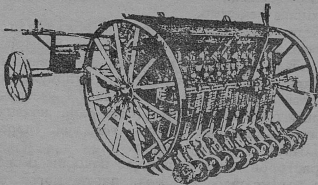
35 серп. Ёглаалөм (комбінірујтөм) көзан Сошныкјас бөр- саыс вөтчөны гөгылјас, көдјас мусө топөдөны.
