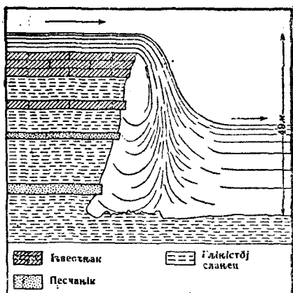
Њагарскёј водопадлөн схема.
