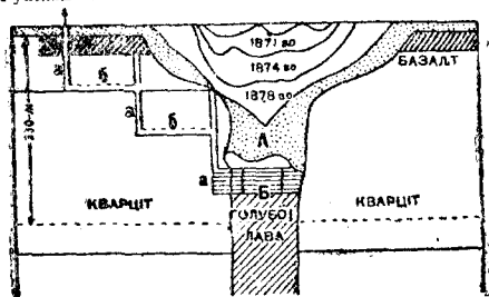
А —Тыртм породажаслн асып а-Шахтажас б-Штрекі б-Пержанін (му пышкын)
