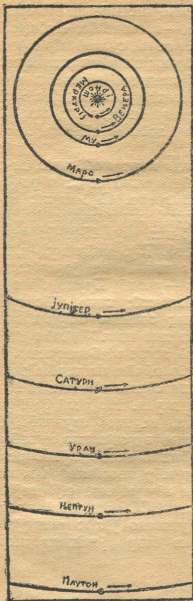
6-öд серпас. Шондi cистема.
