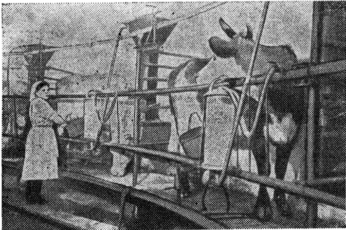
ЧЕЛЯБИНСКОЙ ОБЛАСТЬ. Уйскбй совхозысь Кировскбй отделенбса механизаторьяс лбсьбдбсны лысьтысын установка «карусель». Сийбс монтируйтны отсалбс металлоконструкцияс вбчан Златоустовскбй заводса коллектив. Кьзъ лысьтысын аппарат пунктбма бергалысь платформа вьлб. Кьк часбн позьб лысьтыны 220 мбс. Установка вылын уджалб сбмын нелб морт, центнер йбвлбн себестоимтьыс чинб 25 процент вьлб. СНИМОК ВЬЛЫН: уджалб лысьтысысь мастер А. Е. Давыдова. ТАСС-лбн Фотохроника.
