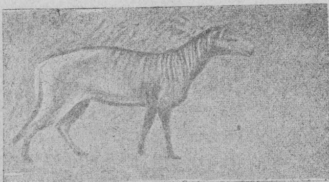
Бөвлөн предокыс.
