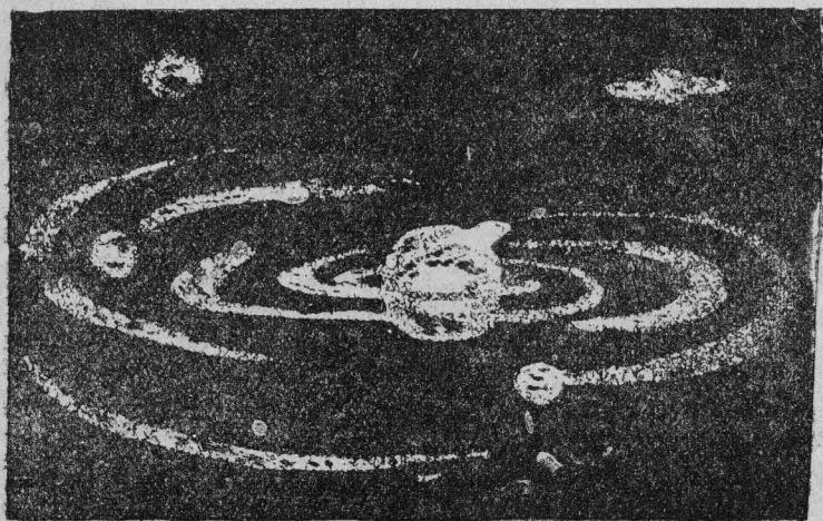
Солнечнөй сiстема артмөм.
