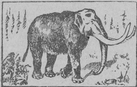
Мамонт.
