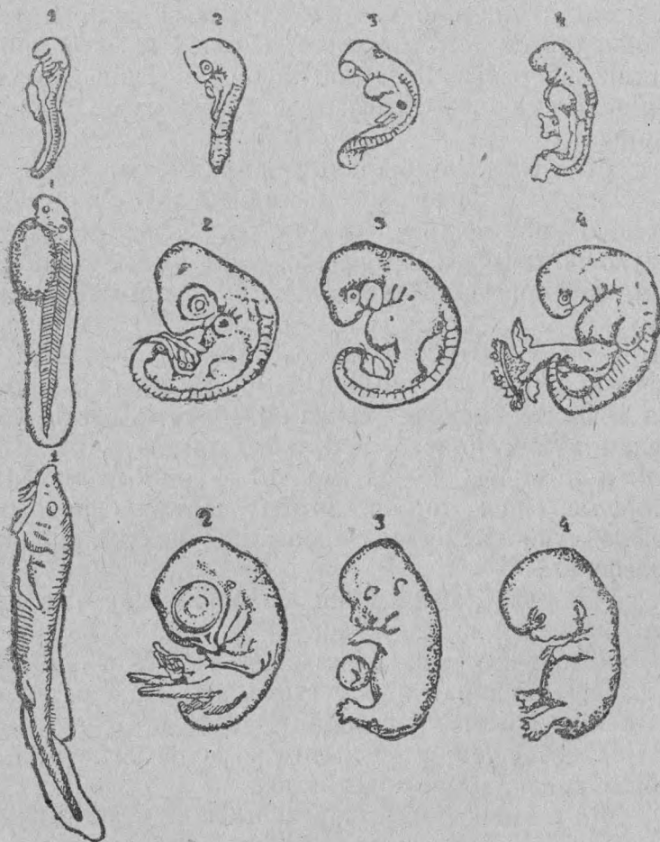
Кызӧ мам кынӧмын быдмӧвы: 1) черӧ зародыш; 2) крошкӧ зародыш; 3) облычана зародыш да 4) морт зародыш.
