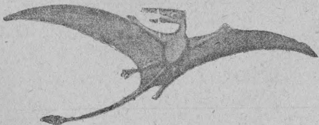
Лебалыс јашцер.
