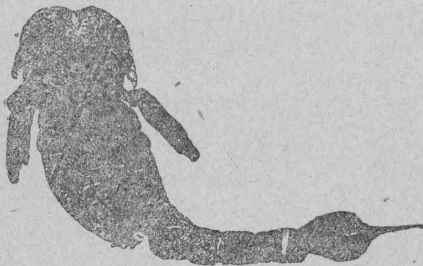
Важја ракообразнӧй.
