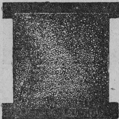
Козув чукёр.
