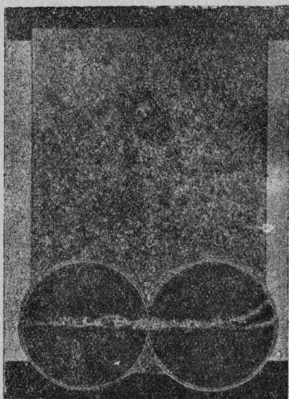
Млечнöј туј.
