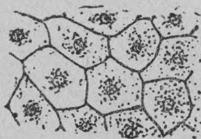
Клеткајас.
