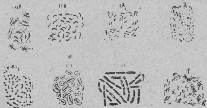
Бактеріјас: I туберкулөздөһ, II сөбүрә јазвалөһ, III тм восһәмәтчан вёсмөһлөһ, IV чумалөһ, V дифтерөјәлөһ, VI холерәсөһ, VII брушһөј тифлөһ. Ставыс јона ыждөдөһа
