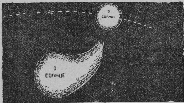
Спиральнөй туманност артмөм.
