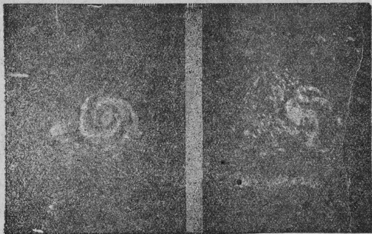
Спiральнöј туманностјас.
