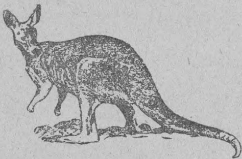
Кенгуру.
