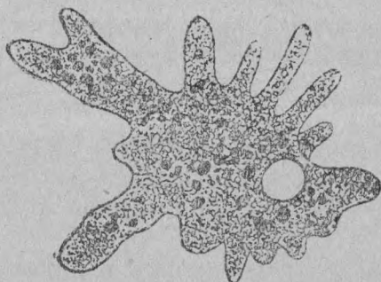
Амеба.
