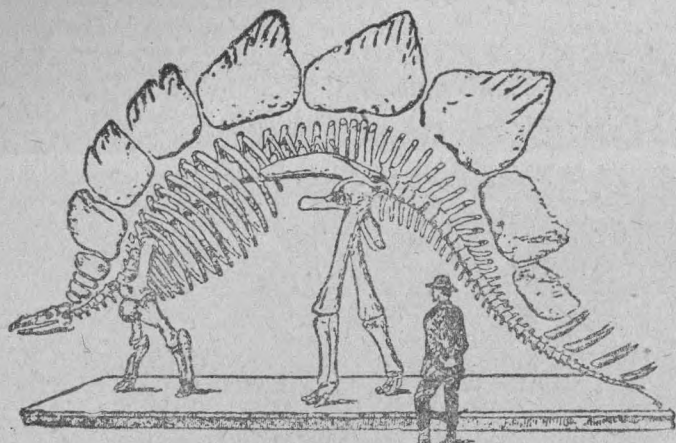
Стегаврлөн костак.
