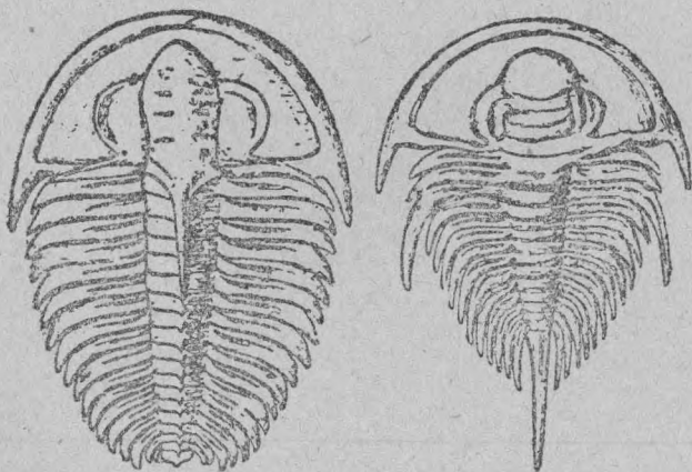
Трїлобїтјас (окам-пелостт).
