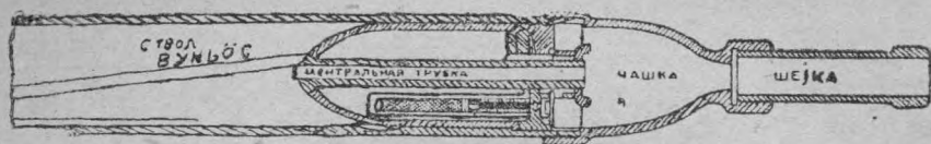
14-d. серпас. Ружејнөј граната мортіркаын
