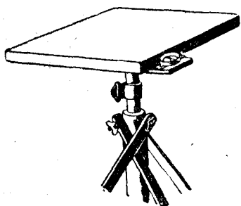
11. Мензула.
