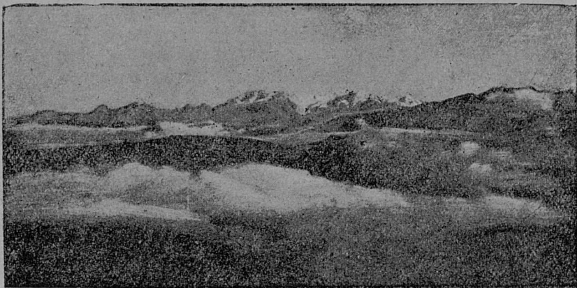
16-õд серпас. Главнõй Кавказскõй хребетлõн серпас. Улиас—ущелјејасын кымõрјас.
