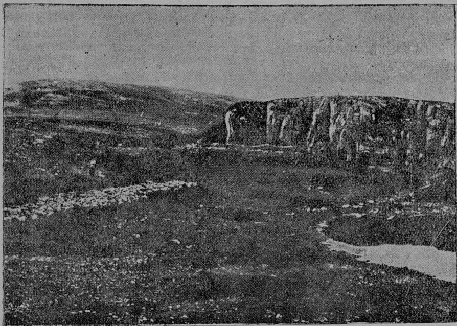
38-ѳд серпас. Јајлалѳн вѳртѳм веркѳсыс ізвестнакјас ердалѳмнјасѳн.
