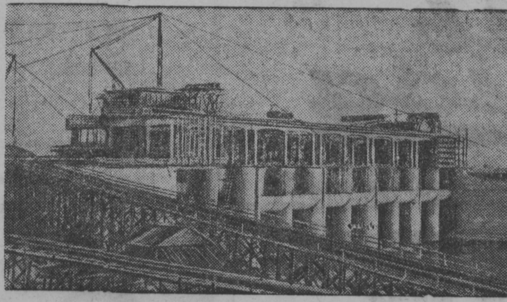
2-д №-а Железобетонной плотинабн общöй вид (Рыбинской гидроузел).
