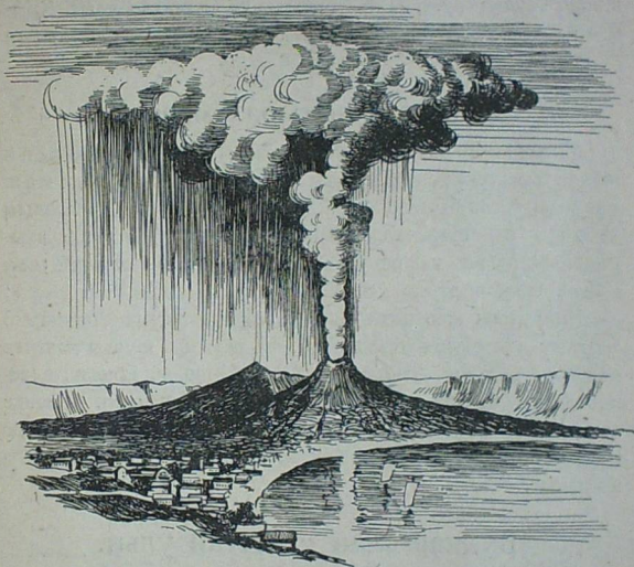
20 сур. Италийыштэ улшо Везувий вулкан.
