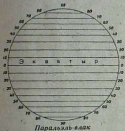
12 сур. Паральэль да мэридиан-влак.
