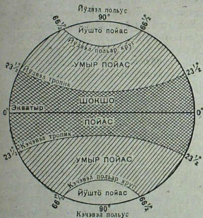
27 сӱр. Мландӧ шарын климыт пойас-влак.
