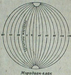
12 сур. Паральэль да мэридиан-влак.
