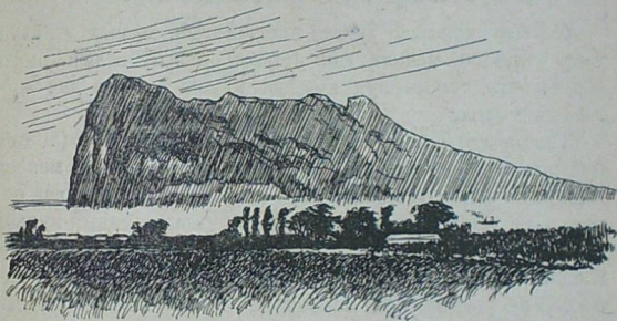
21 сүр. Гибралтар пролив. Гибралтарын Йэвроп вэл кў сэржэ.
