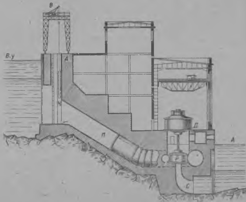
103 сур. Гидроэлектро станцилэн лэсьтэмез.
