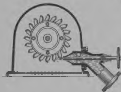
99 сур. Пельтонлэн турбинаэз.
