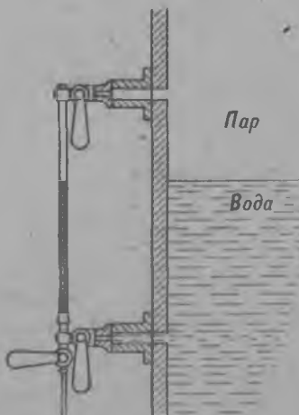
77 сур. Паровой пуртылэн ву мертан пиалазэ.
