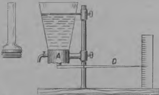
84 сур. Кизер макеослэн пыдэсо зйбемзы посудалэн тусэзлэсь уг поты, посуда тус'я уг вош'яськы.
