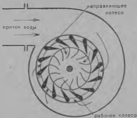
102 сур. Фрэнсислэн турбинааз.
