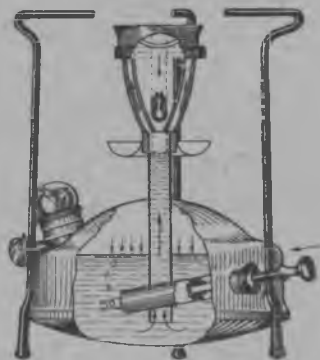
118 сур. Примус.
