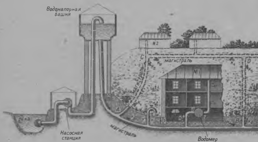
104 сур. Кар водопроводлэн схемаэз.
