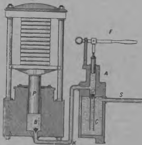
72 сур. Гидравлической пресслэн схемаэз.
