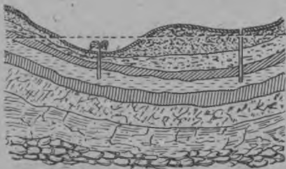
78 сур. Артезиан колодча
