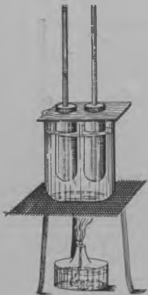
44 сур. Кизер макеослэсь паськытамзэс ёшотон.
