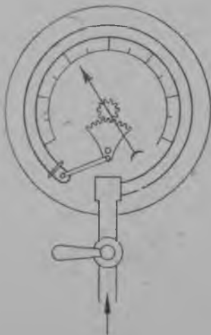
117 сур. Манометр.
