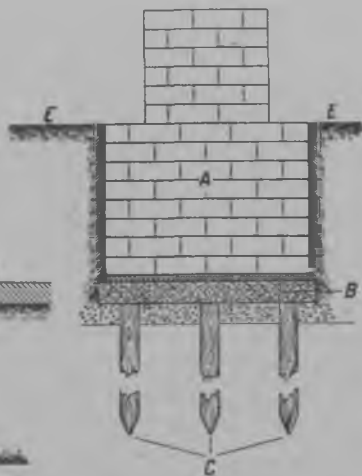
64 сур. Бетон миндэр'ёс вылэ пуктэм фундамент. Грунт пуктос'ёсын юнматэмын. Кузь пуктос'ёс пум'ёсынызы гинэ возьматэмын.
