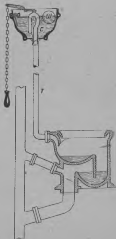
106 сур. Сёросысь мисьтйськонлэн лэсьтэмез.
