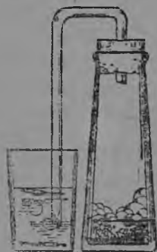
46 сур. Углекислой газ поттон.
