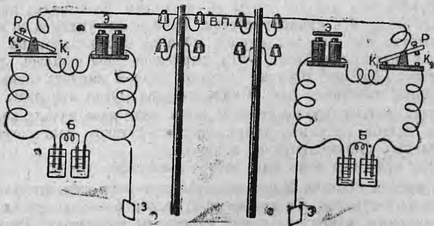
Кызы телеграф ужа.
