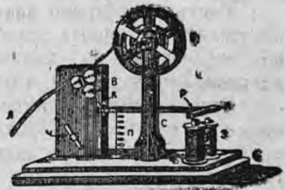
Телеграфлэн аппаратэс.
