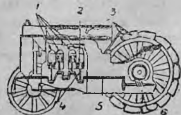
1) Цилиндр. 2) Поршень. 3) Карасин бак. 4) Поршень выд. 5) Коленчатый вал.
