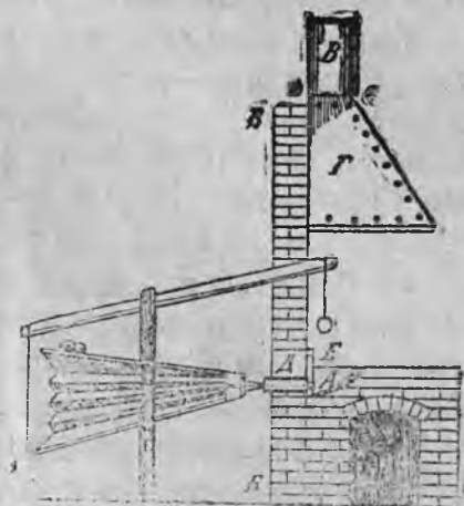
А — эгыр суроп, корт пёсатоп. Б — стена. В — чын кыскон труба. Г — колпак. Д — омыр пьрон.
