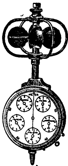
104 суред. Чашеч- ной вукоен анемо- метр.
